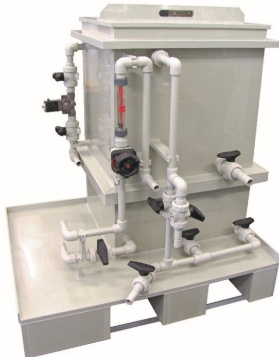
Mobiler Apparat im Bereich Galvanotechnik, hergestellt aus Polypropylen
